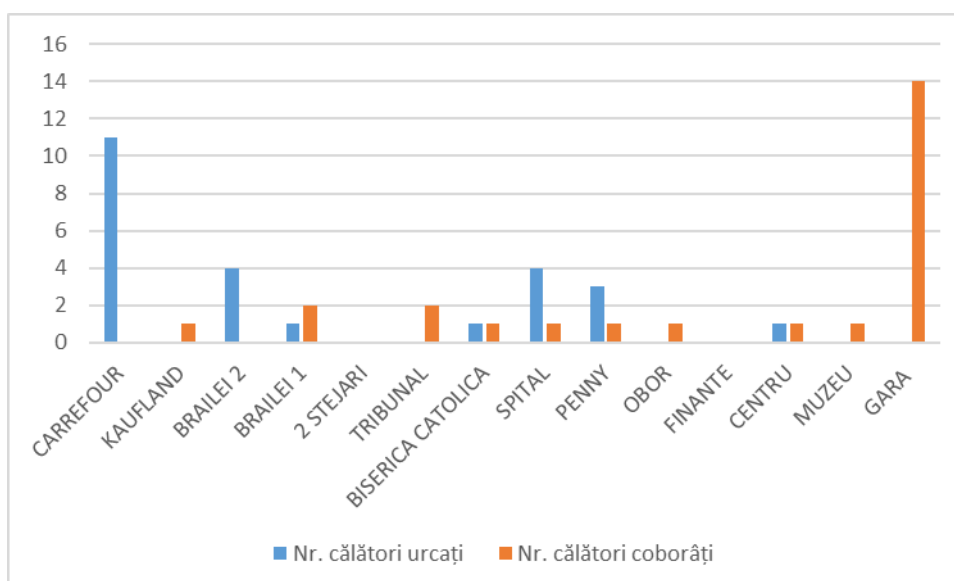
Fig. 3.100. Număr călători urcați / coborâți - Traseul 7 Retur - PM
