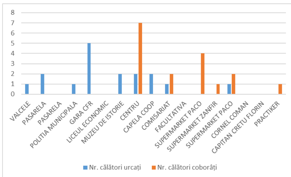
Fig. 3.90. Număr călători urcați / coborâți - Traseul 51 Tur - AM
