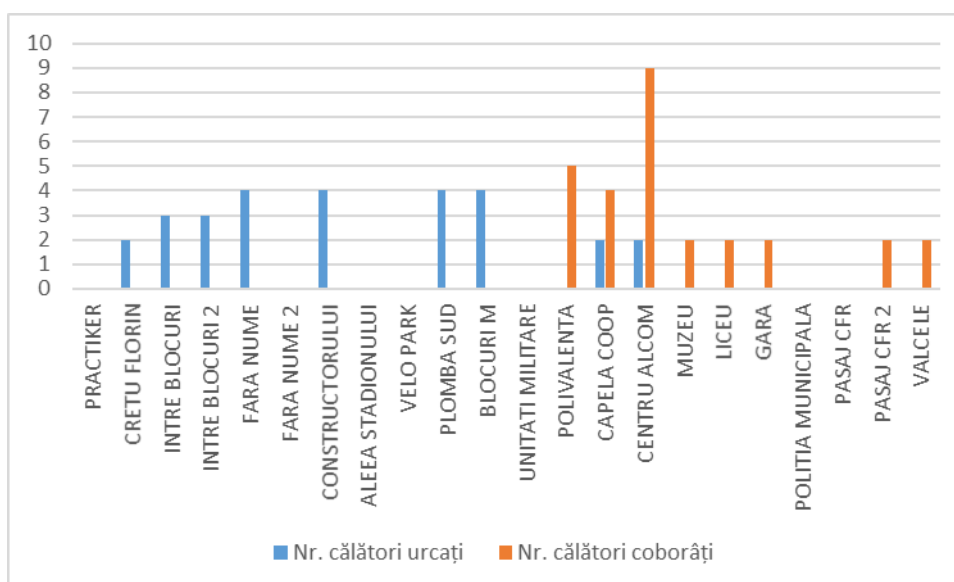
Fig. 3.93. Număr călători urcați / coborâți - Traseul 51 Retur - AM
