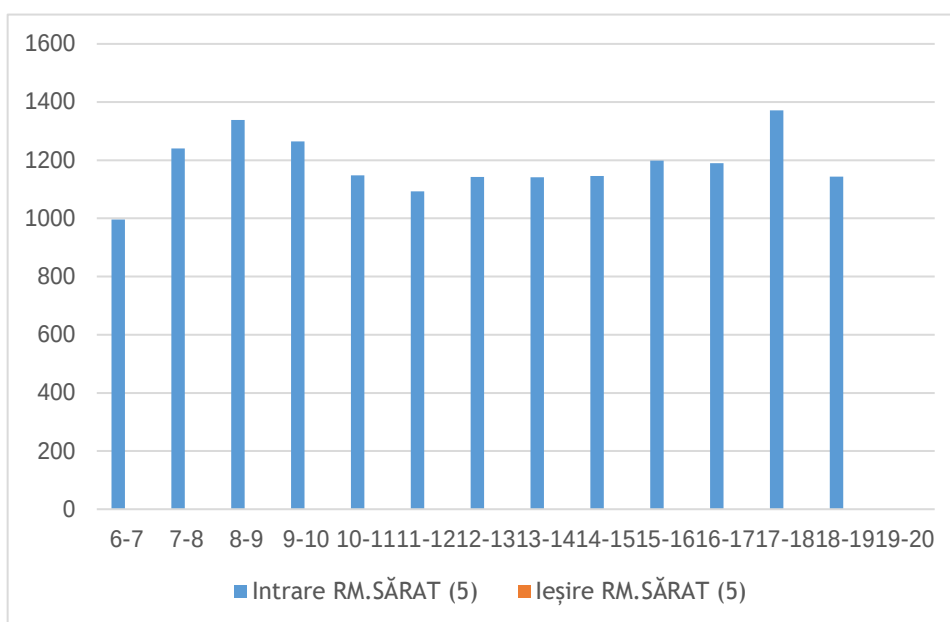
Fig. 3.60. Variația fluxului de trafic, Intrare Râmnicu Sărat Sud
