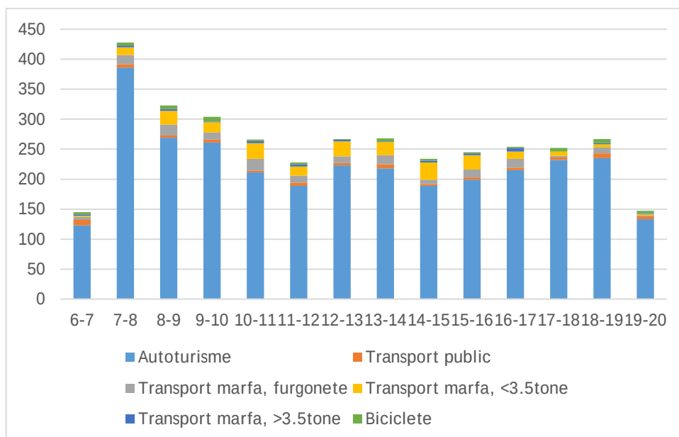
Fig. 3.67. Variația fluxului de trafic pe tipuri de vehicule, Intrare Vîlcelele Nord-Vest
