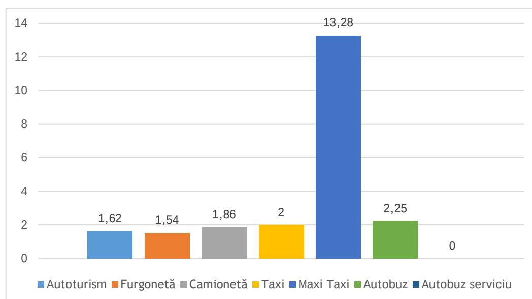
Fig. 3.70. Grad de umplere, Intrare Vâlcelele Nord-Vest
